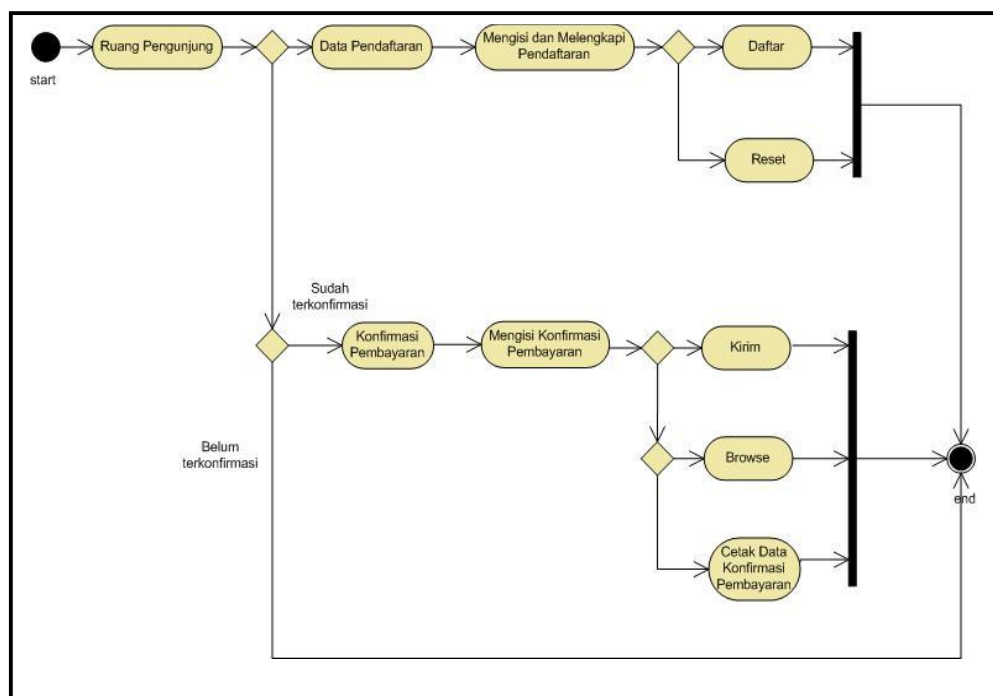
Gambar IV. 4 Activity Diagram Halaman Pengunjung dan Peserta
