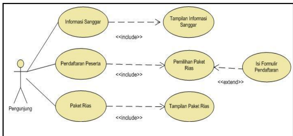
Gambar IV. 1 Use Case Pendaftaran Online pada Halaman Pengunjung
