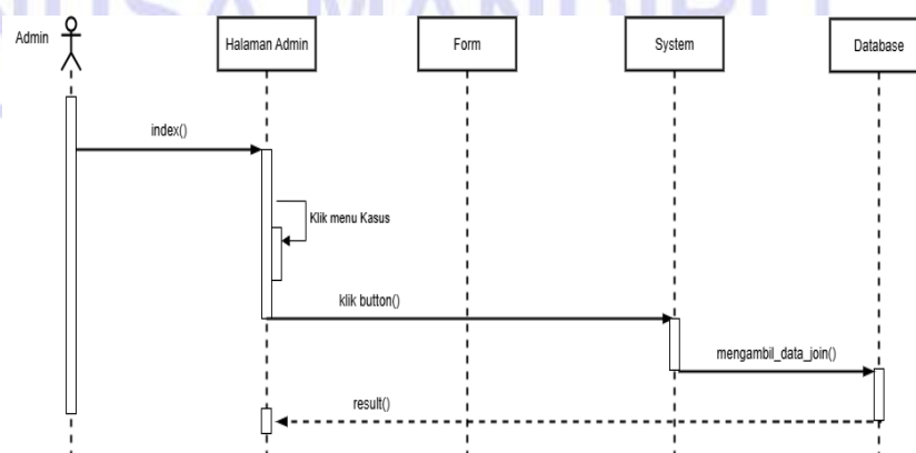
Gambar IV.23 Sequence Diagram Admin Melihat Data Kasus
