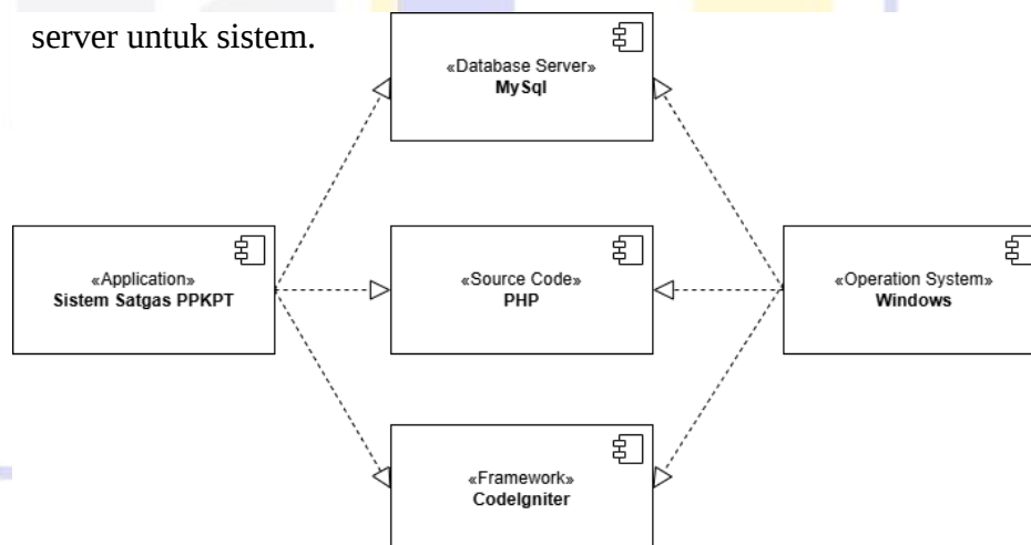
Gambar IV.34 Component Diagram Sistem Web Satgas PPKPT
