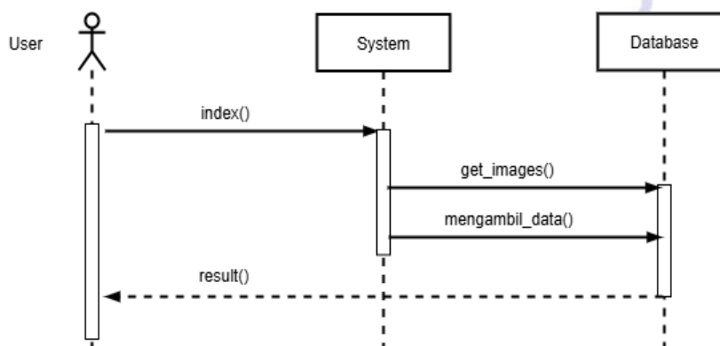
Gambar IV.20 Sequence Diagram User Melihat Informasi Kegiatan dan Berita
