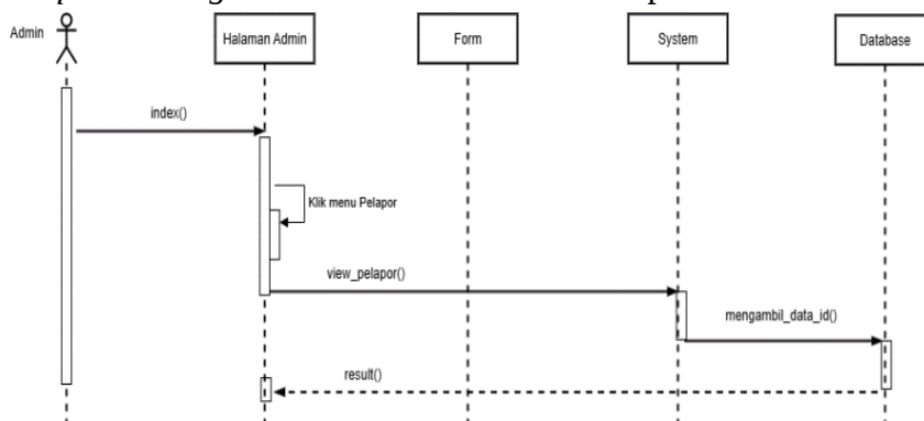
Gambar IV.24 Sequence Diagram Admin Melihat Data Pelapor
