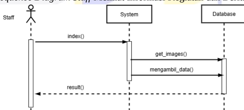
Gambar IV.29 Sequence Diagram Staff Melihat Informasi Kegiatan dan Berita
