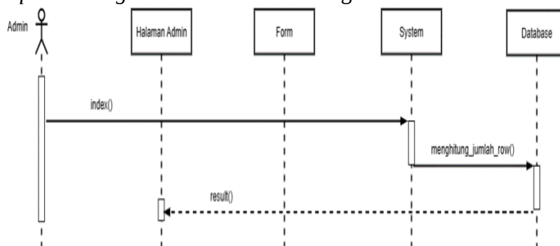
Gambar IV.27 Sequence Diagram Admin Melihat Ringkasan Statistik
