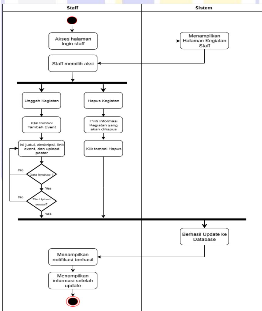
Gambar IV.11 Activity Diagram Kelola Informasi Kegiatan
