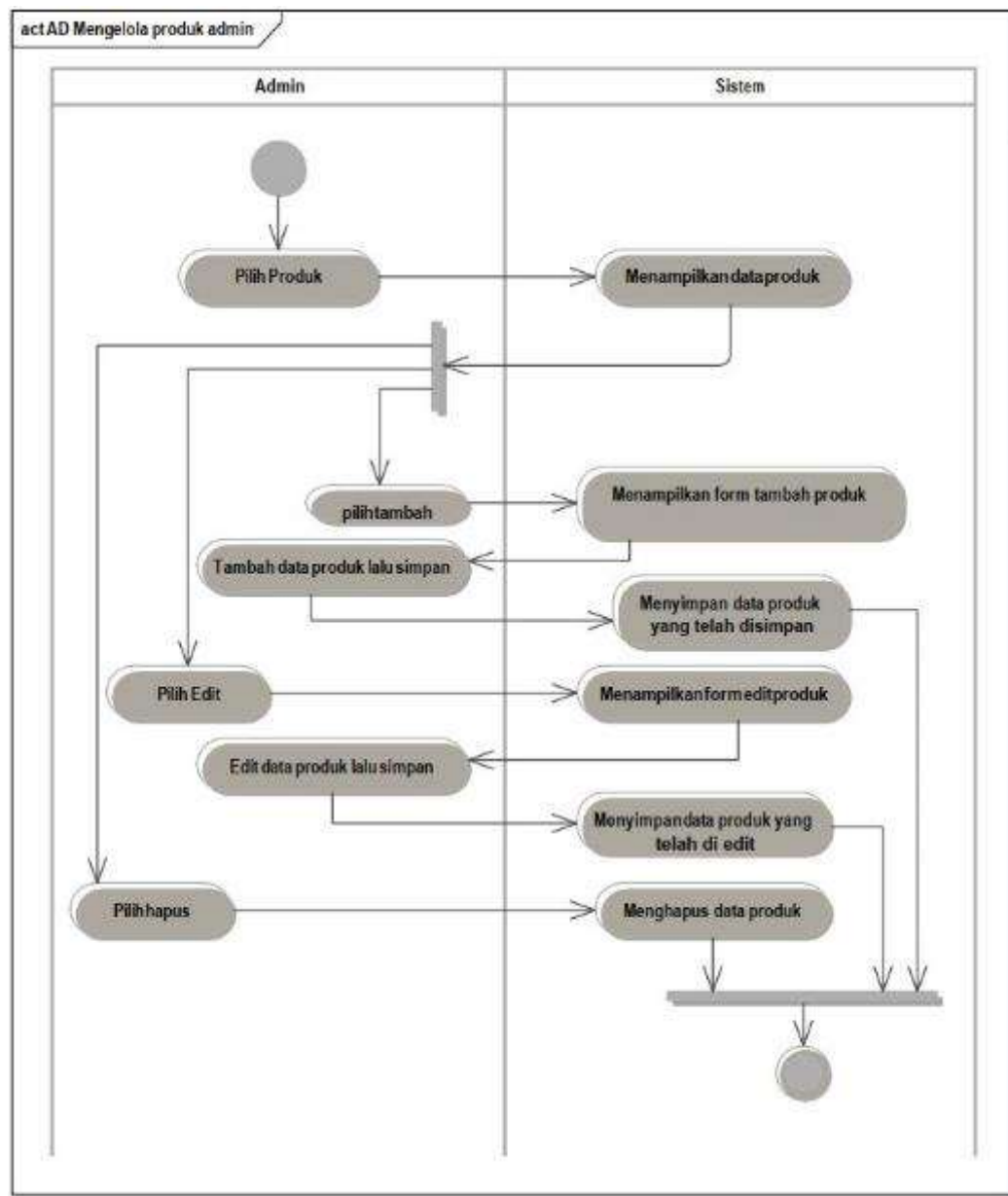
Gambar 14. Activity Diagram Kelola Produk
