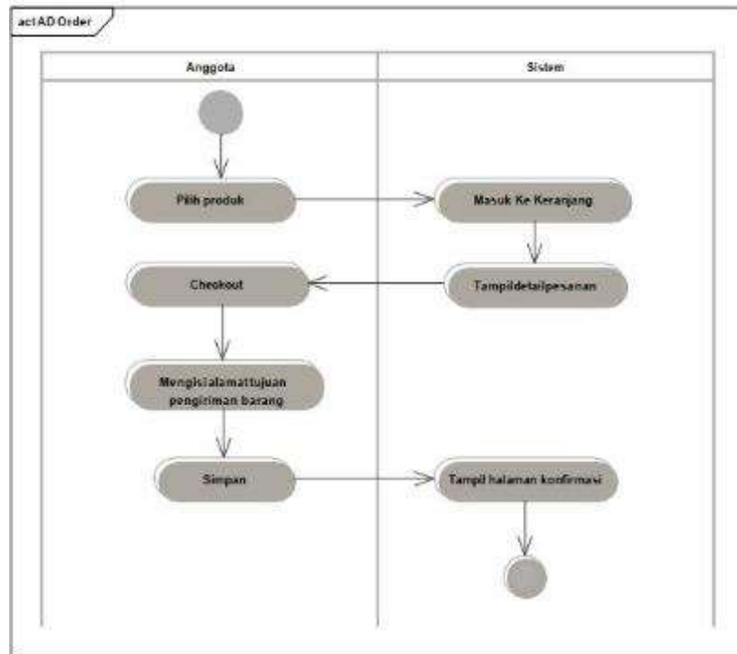
Gambar 7. Activity Diagram Pemesanan
