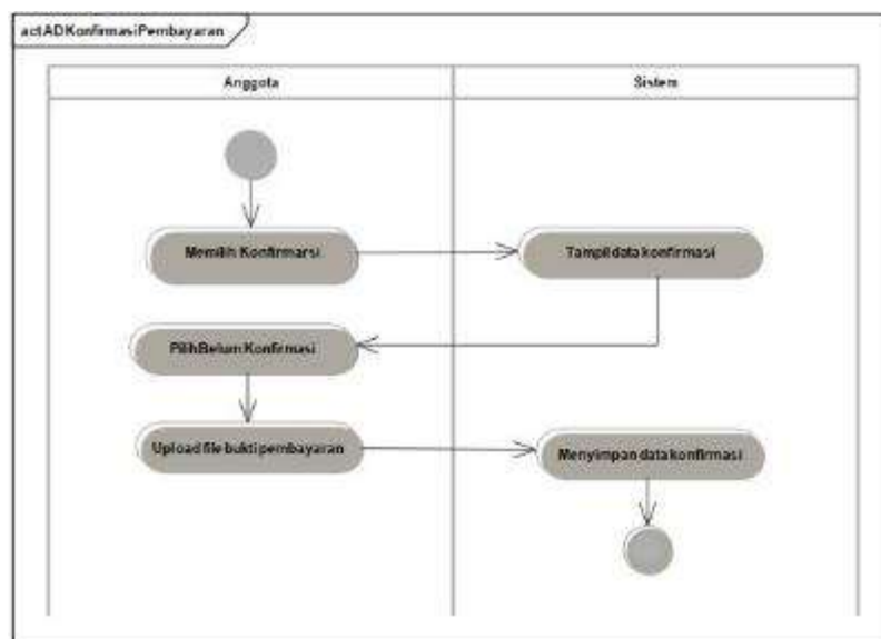
Gambar 8. Activity Diagram Konfirmasi Pembayaran
