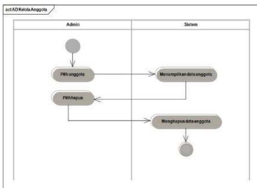
Gambar 17. Activity Diagram Kelola Anggota
