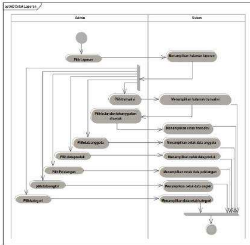
Gambar 20. Activity Diagram Cetak Laporan
