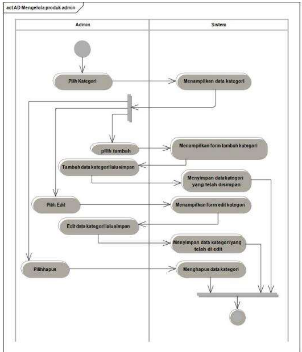
Gambar 14. Activity Diagram Kelola Kategori
