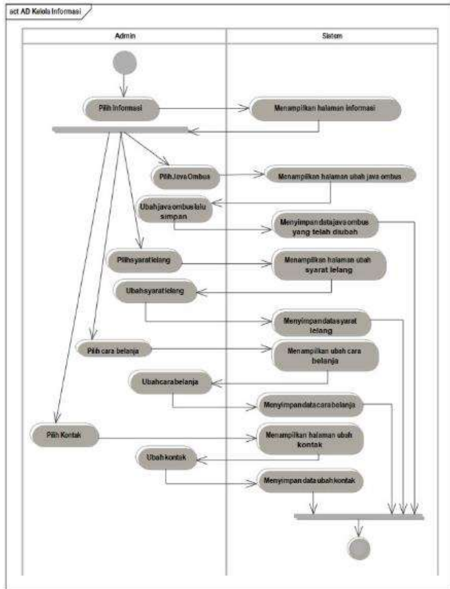
Gambar 19. Activity Diagram Kelola Informasi
