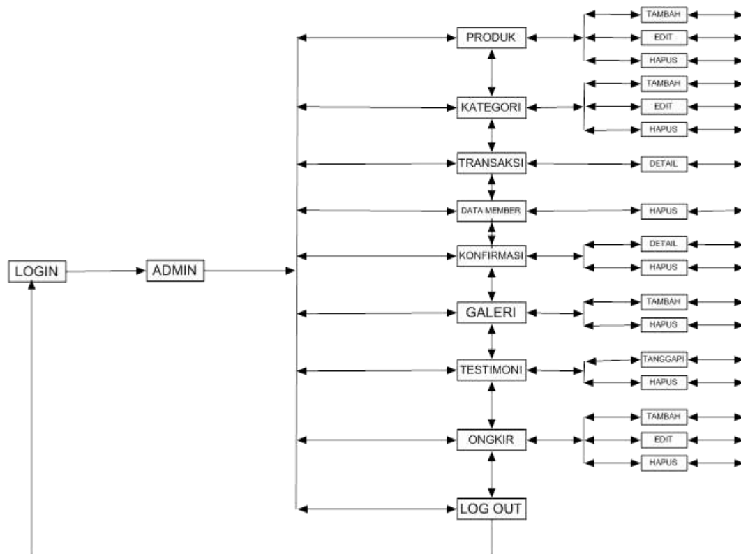
Gambar III.5. Struktur Navigasi Halaman Index Admin
