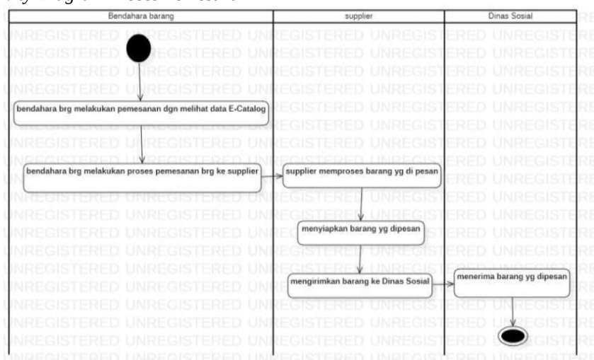
Gambar 3 Activity Diagram proses pemesanan
