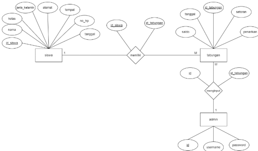
Gambar 4. ERD Sistem Pengolahan Tabungan Berbasis Web
