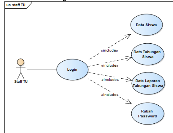
Gambar 2. Use Case Diagram pada Sistem Usulan
