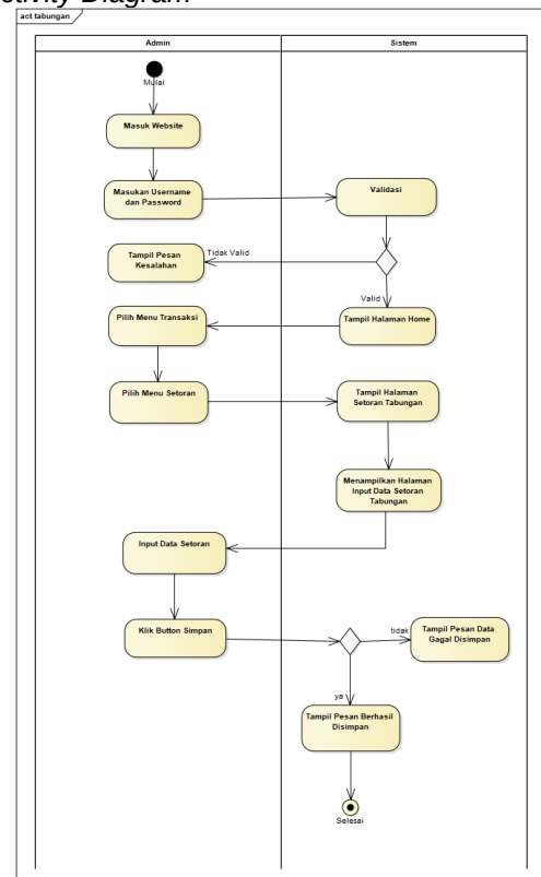
Gambar 3. Activity Diagram pada Website Pengolahan Tabungan
