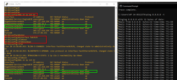
Gambar 14. Mematikan Koneksi ISP 2
