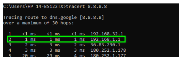
Gambar 13. Traceroute dari laptop user
