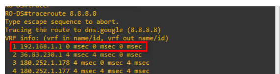
Gambar 12. Trace route dari router
