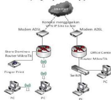
Gambar 3. Topologi Jaringan Usulan
