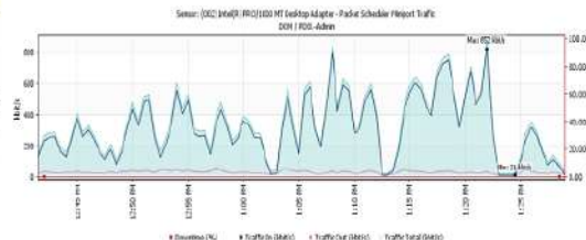
Gambar 15. PD01-Admin pada PRTG sebelum implementasi
