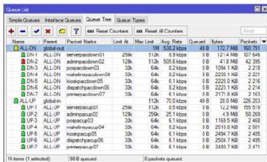
Gambar 21. Queue Download PD01-Admin pada Batas Maksimum
