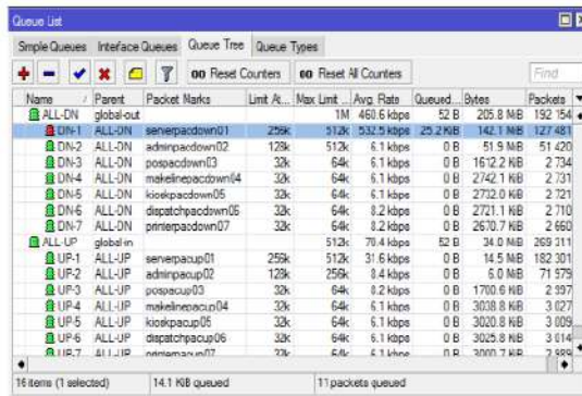
Gambar 20. Queue Download PD01-Server pada Batas Maksimum
