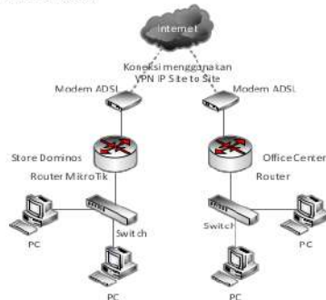
Gambar 2. Topologi Jaringan pada store Dominos Pizza di PT. MAP
