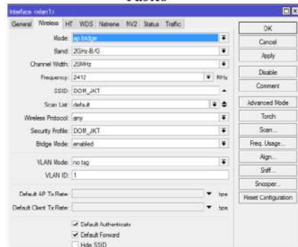
Gambar 12. Menu Wireless pada Interface Wireless
