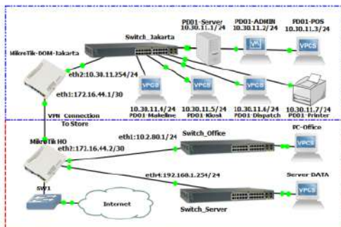
Gambar 4. Skema Jaringan Usulan
