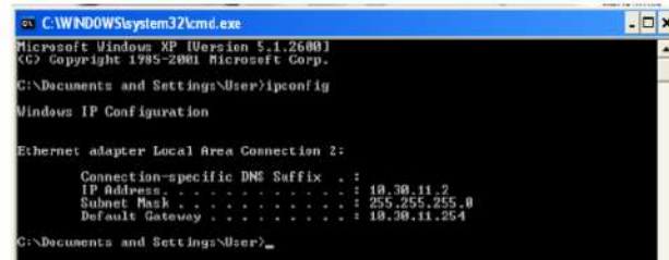
Gambar 13. IP Address pada Komputer PD01-Admin
