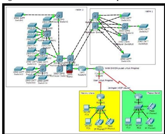
Gambar 2. Pengembangan Topologi Star dan Jaringan WAN
