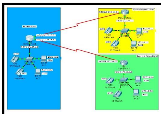
Gambar 3. Skema Jaringan Komunikasi VOIP Usulan pada BKKBN Pusat
