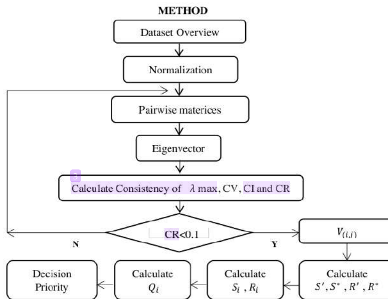
Fig. 1. AHP-VIKOR Algorithm
