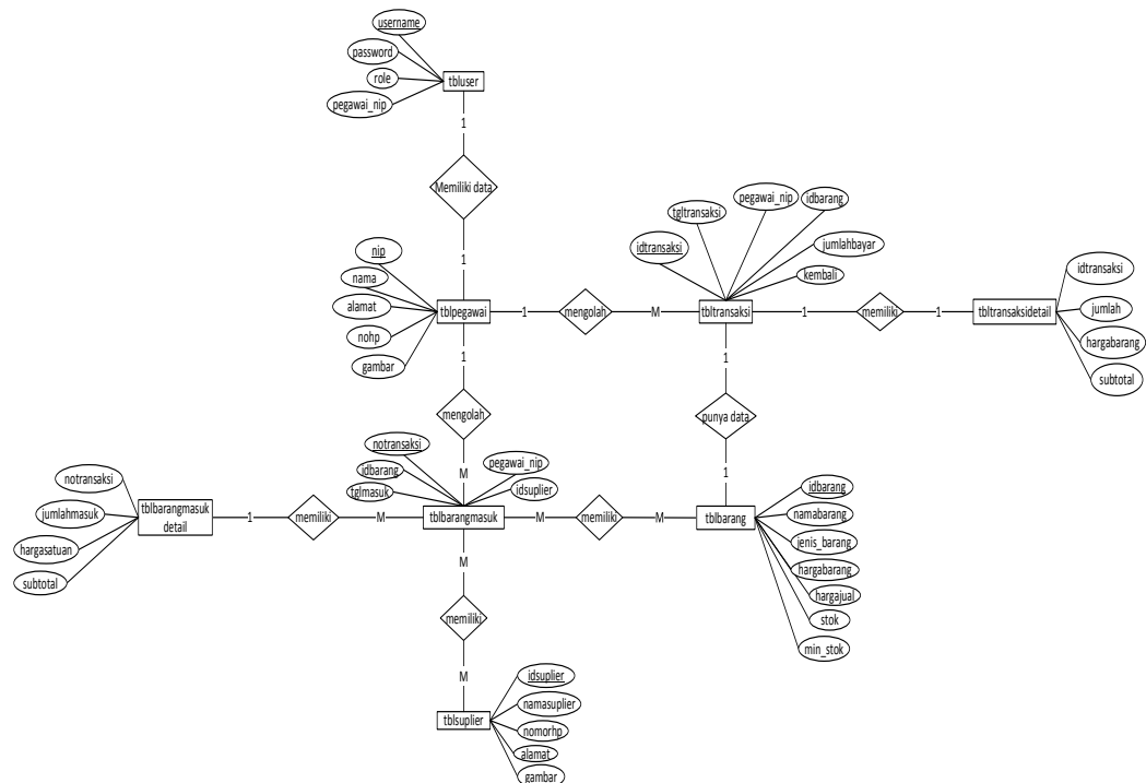
Gambar 1. ERD
