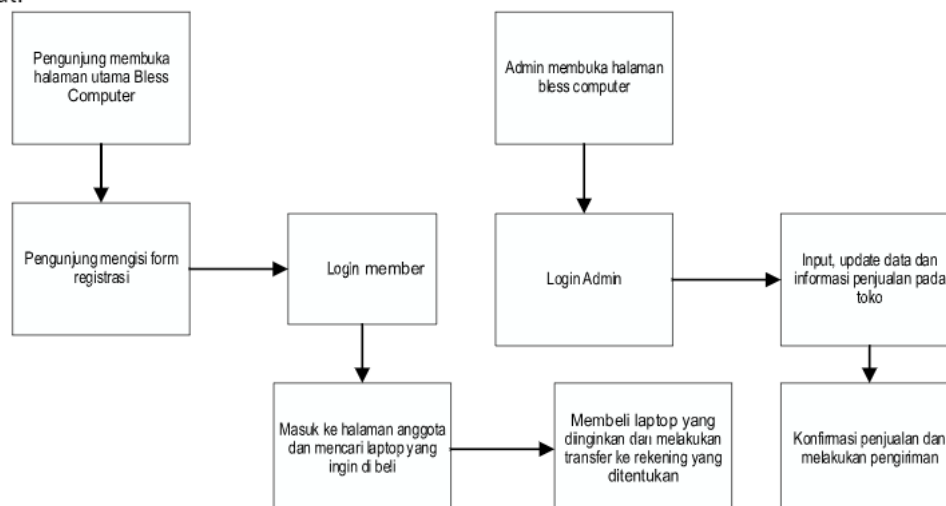
Gambar 3. Urutan Kegiatan Sistem Penjualan Laptop Berbasis Web
