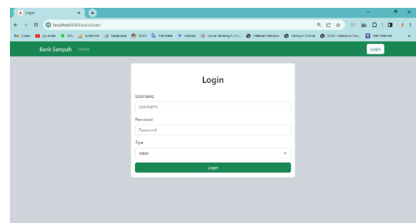
Gambar 7. Halaman Login
