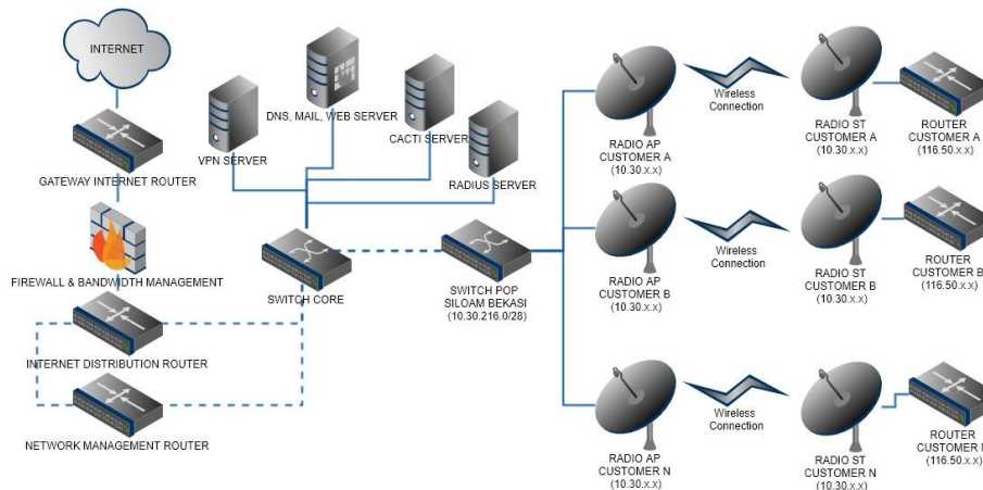
Gambar 2. Topologi Jaringan Berjalan
