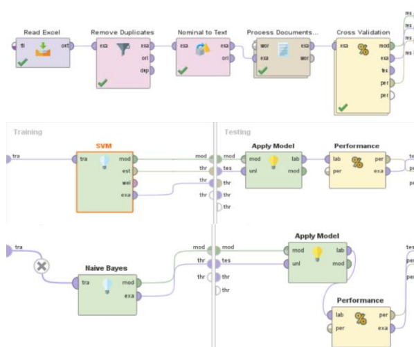
Gambar 4. Desain Model Algoritma (SVM) dan NB
