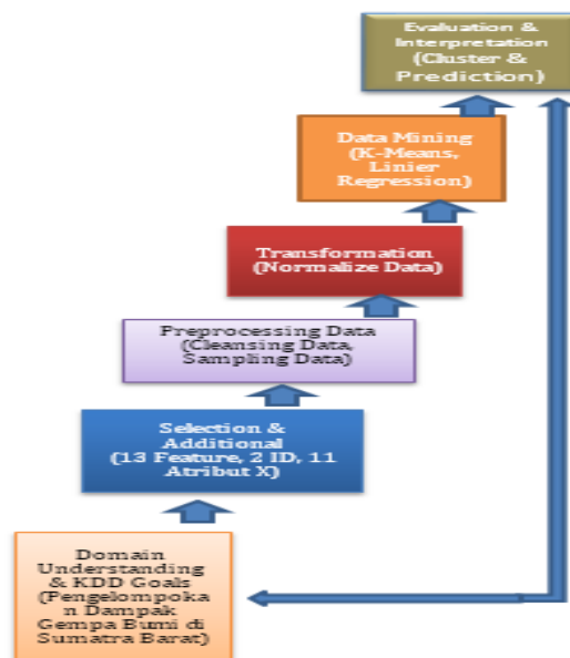
Gambar 1. Model KDD Modifikasi
