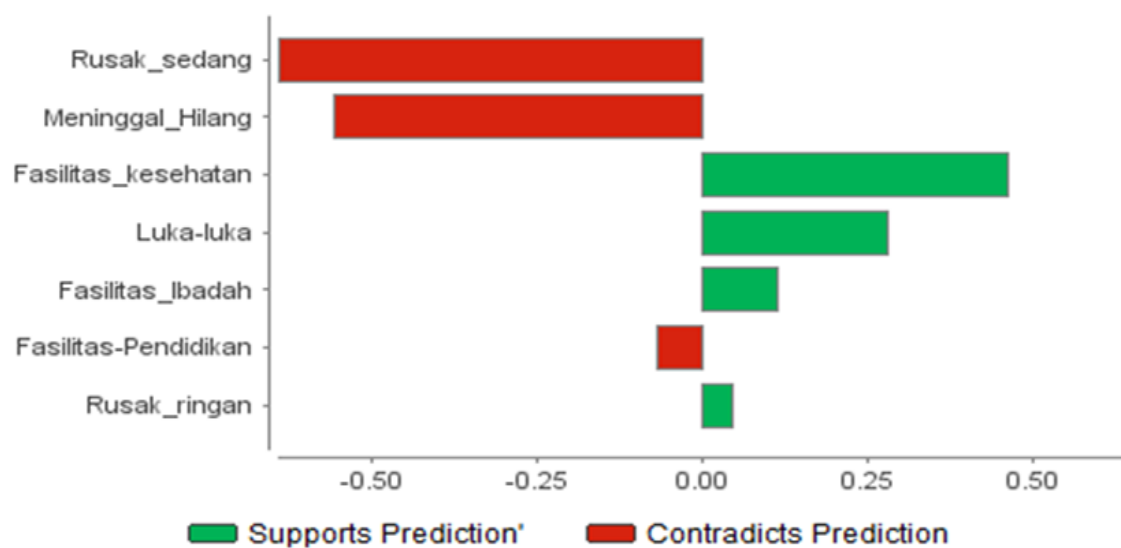
Gambar 4. Hasil Visualisasi Intensitas Dampak Gempa di Provinsi Sumatera Barat.
