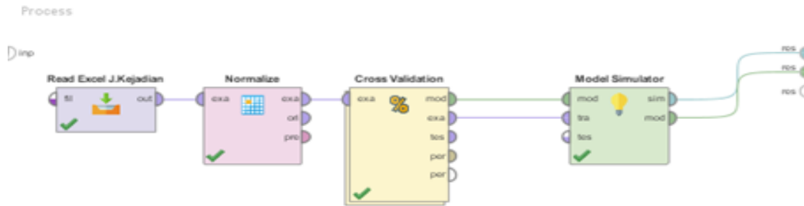
Gambar 3. Model Pengolahan Regresi Dengan Algoritma Linear Regression
