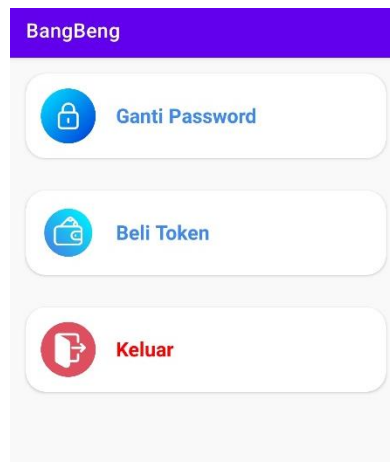
Gambar 14. Halaman Pengaturan
