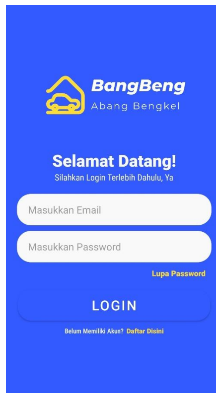
Gambar 1. Halaman Login
