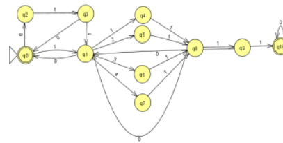
Gambar 3. FSA VM seragam karyawan.
