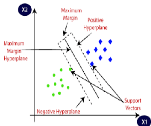
Gambar 5. Algoritma SVM
