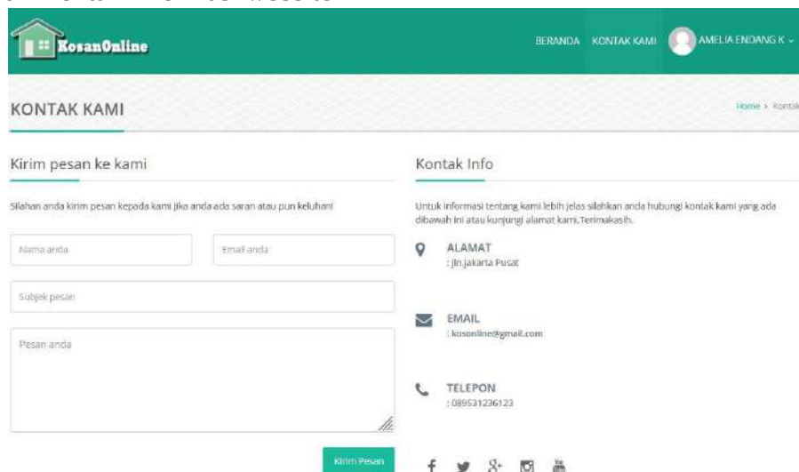
Gambar 6. Kontak Kami
