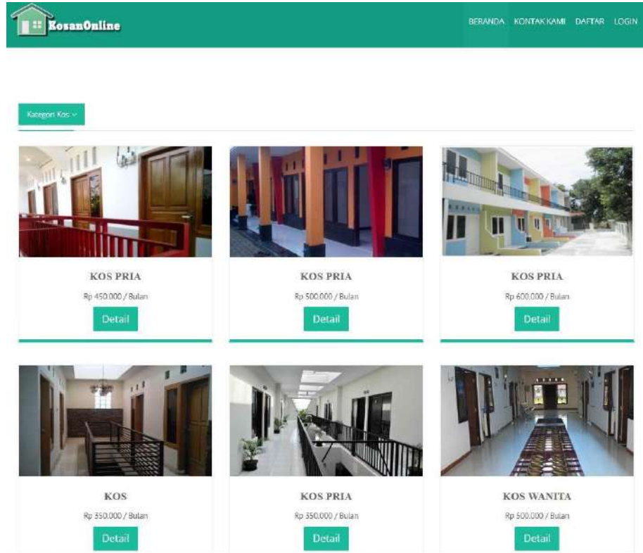
Gambar 1. Menu Awal
