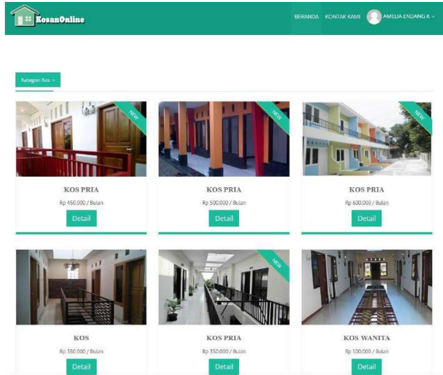
Gambar 5. Menu Beranda
