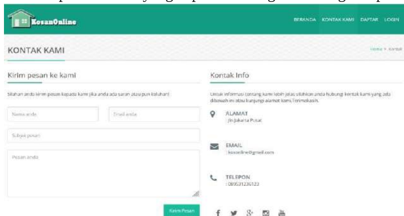
Gambar 2. Menu Kami
