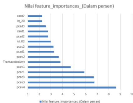
Gambar 3 Feature Importance Score Paling tinggi pada model dasar
