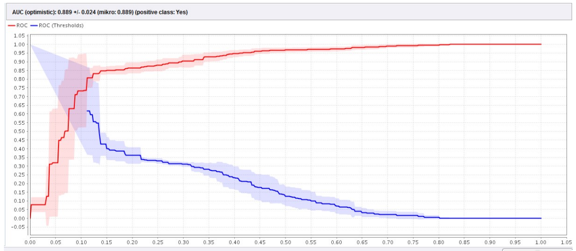
Gambar 4.6 Nilai AUC dalam grafik ROC Algoritma C4.5 Berbasis PSO
