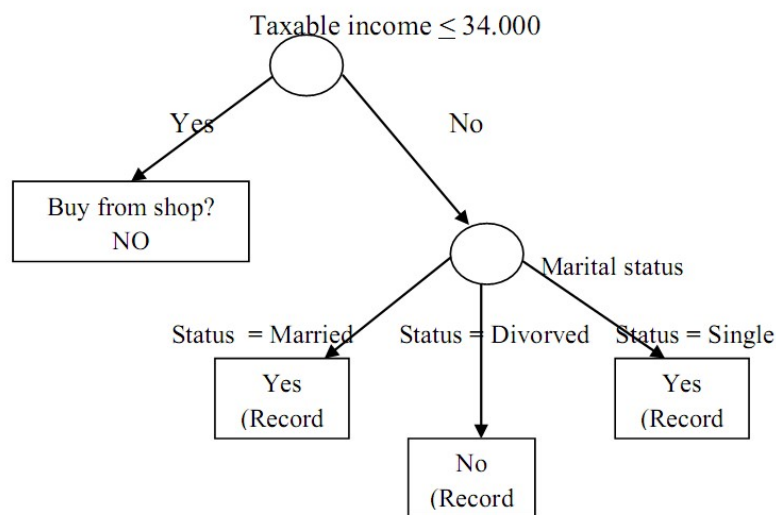
Gambar 2.1 Contoh konsep pohon keputusan sederhana (Gorunescu, 2011)
