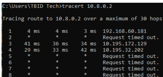
Gambar 37. Hasil Tracert Tanpa VPN
