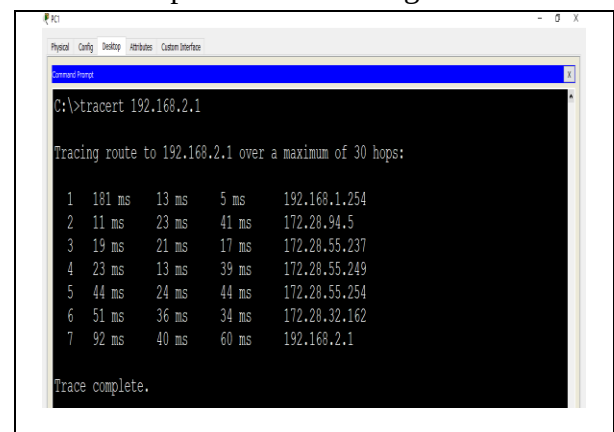
Gambar 10 Pengujian Jejak Koneksi Client Kantor Pusat ke Client Kantor Cabang dengan ISP Pertama Down
