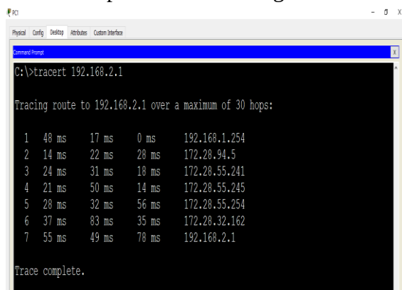
Gambar 8. Hasil Pengujian Jejak Koneksi Client Kantor Pusat dengan Client Kantor Cabang dengan 2 ISP Active
