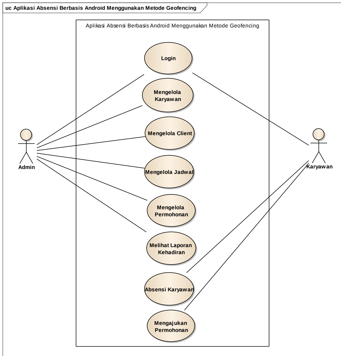
Gambar 1 Use Case Diagram Aplikasi Absensi Berbasis Android Menggunakan Metode Geofencing
