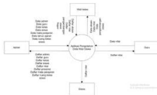
Gambar 1: Diagaram Konteks
