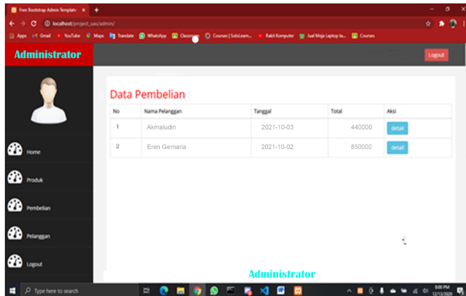
Gambar 6. Menu pembelian
