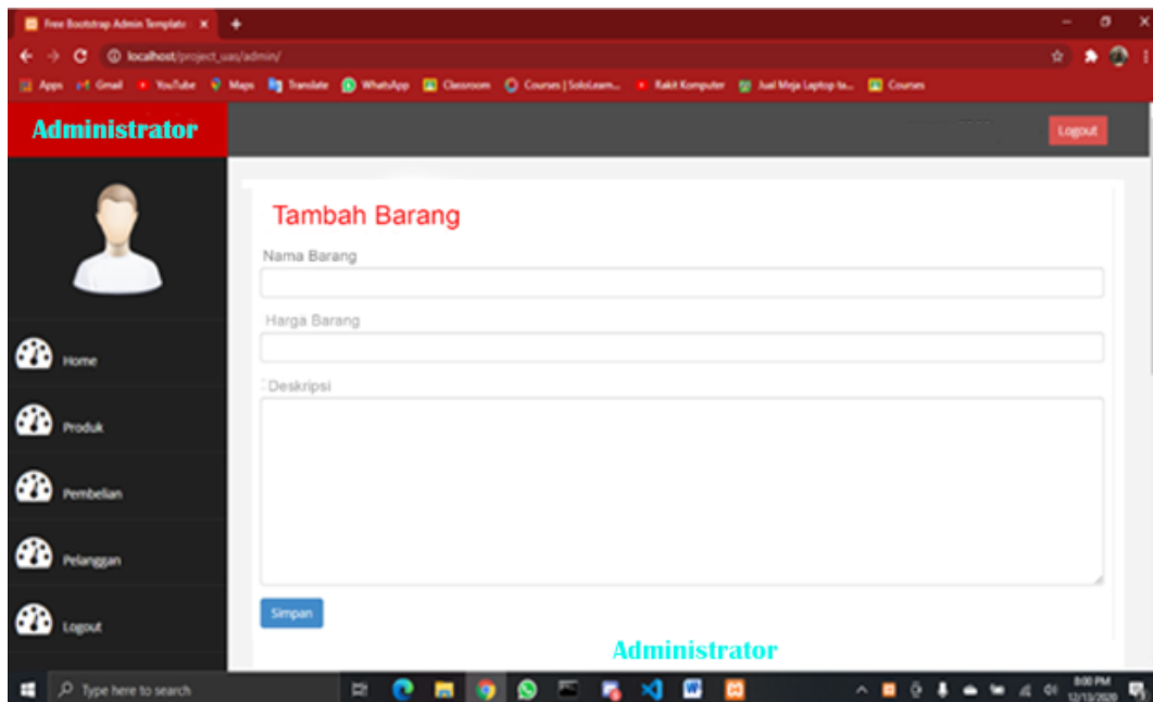
Gambar 4. Tambah Barang
