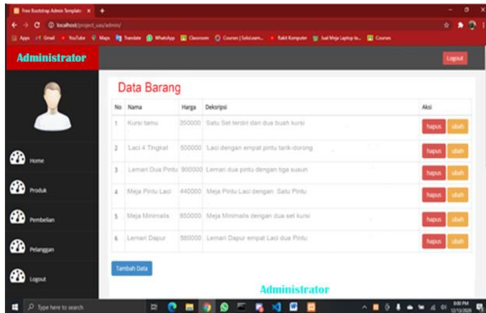
Gambar 3. Data Barang
