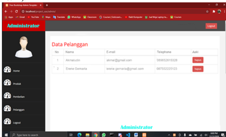
Gambar 2. Data pelanggan
