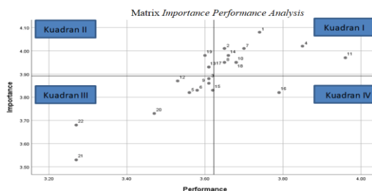
Gambar 1 Diagram Kartesius evaluasi website BPJS Kesehatan
