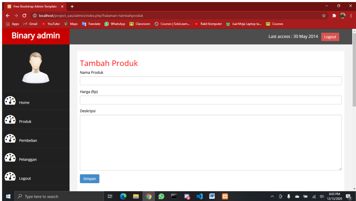
Gambar 4. Tambah produk
