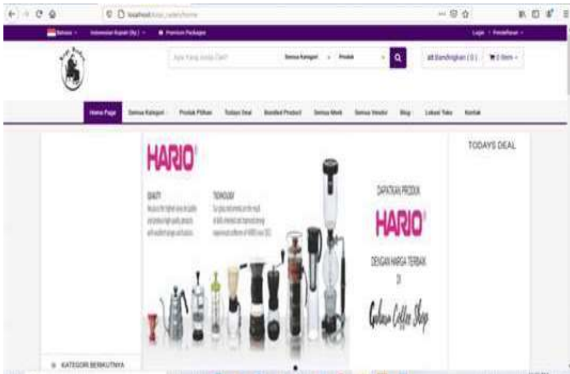
Gambar 1. Menu Utama
