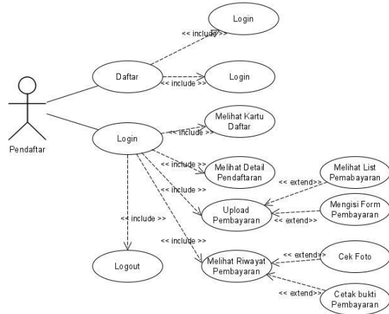
Gambar 3. Use case diagram pendaftaran
