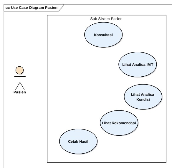
Gambar 3. Use Case Diagram User (Pasien)
