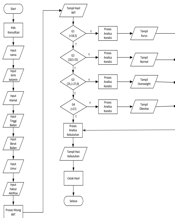
Gambar 1. Algoritma Pakar
