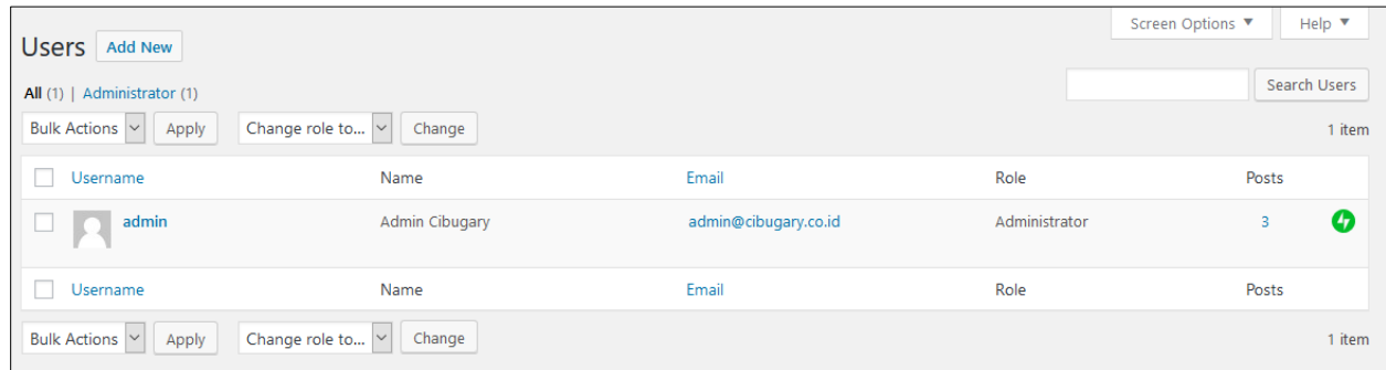
Gambar 3. Data pengguna/users.
