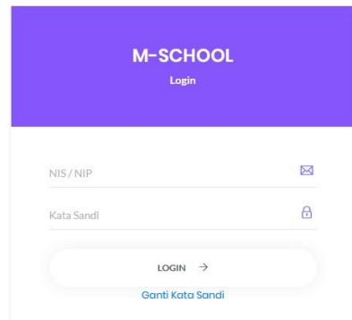
Gambar 2 Halaman Login
