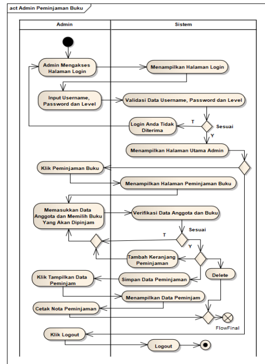
Gambar 3. Activity Diagram Peminjaman Buku
