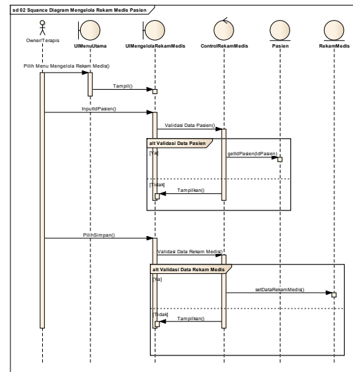
Gambar 5 Squence Diagram Mengelola Data Rekam Medis
