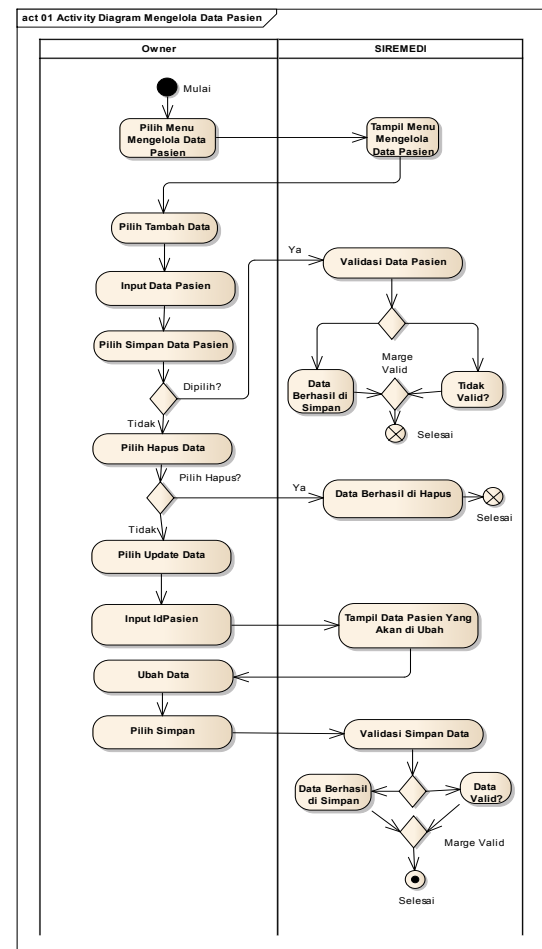
Gambar 2 Activity Diagram Mengelola Data Pasien
