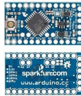
Figure 1. Arduino Pro Mini
