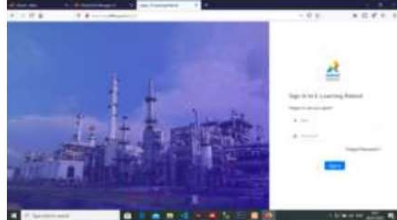
Gambar 4. Halaman Login
