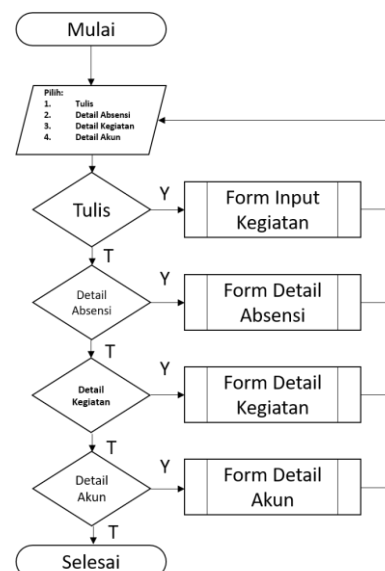
Gambar 11 Flowchart Menu Utama
