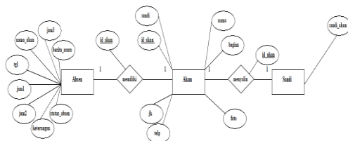
Gambar 8 ERD Aplikasi Abang 1.0
