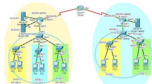
Gambar IX Pengujian Jaringan Akhir Access Inter-VLAN
