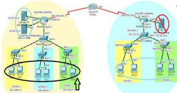
Gambar X. Pengujian Jaringan Akhir Kantor Utama
