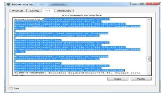
GambarII. Membuat Interface port Inter-Vlan pada Router
