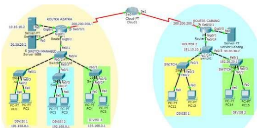
Gambar1. Skema Jaringan
