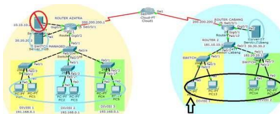
Gambar XII Pengujian Jaringan Akhir Kantor Cabang
