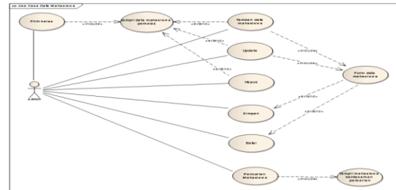
Gambar 3. Use Case Diagram Halaman Admin Mengelola Data Mahasiswa
