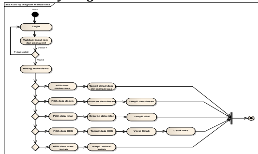
Sumber: (Sastra et al., 2019) Gambar 6. Activity Diagram Mahasiswa
