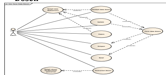
Gambar 4. Use Case Diagram Halaman Admin mengelola Data Dosen
