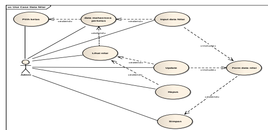
Gambar 5. Use Case Diagram Halaman Admin Mengelola Data Nilai
