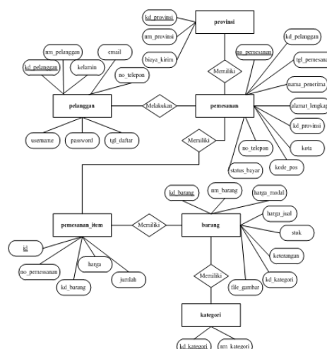
Gambar 8. Rancangan ERD Sistem Penjualan Sparepart motor.
