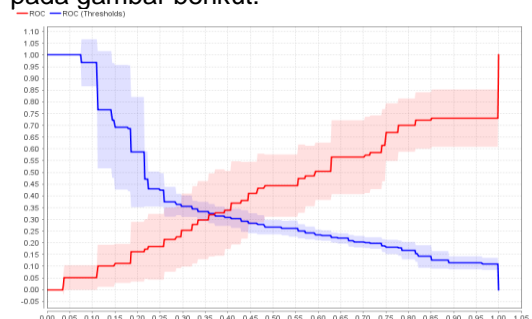
Gambar 16. AUC Algoritma C4.5
