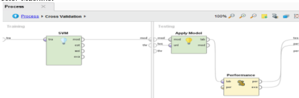
Gambar 6. Layout Proses Support VectorMachine dengan 10-Fold Cross Validation.
