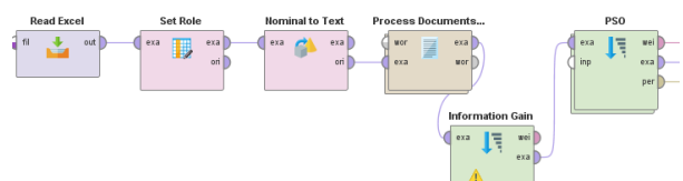
Gambar 13. Operator PSO dalam proses
