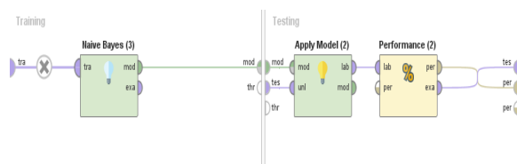
Gambar 10. Bagian dalam Cross Validation
