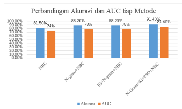
Gambar 13. Grafik perbandingan hasil Akurasi dan AUC
