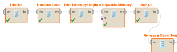
Gambar 7. Penggunaan operator N-gram di RapidMiner
