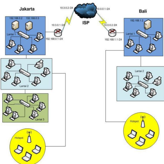
Gambar 2. Topologi VPN kantor pusat dan cabang
