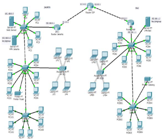
Gambar 3. Skema jaringan usulan
