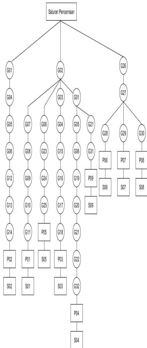
Gambar 1, Pohon Keputusan
