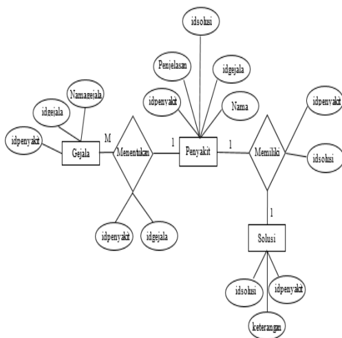
Gambar 2. ERD
