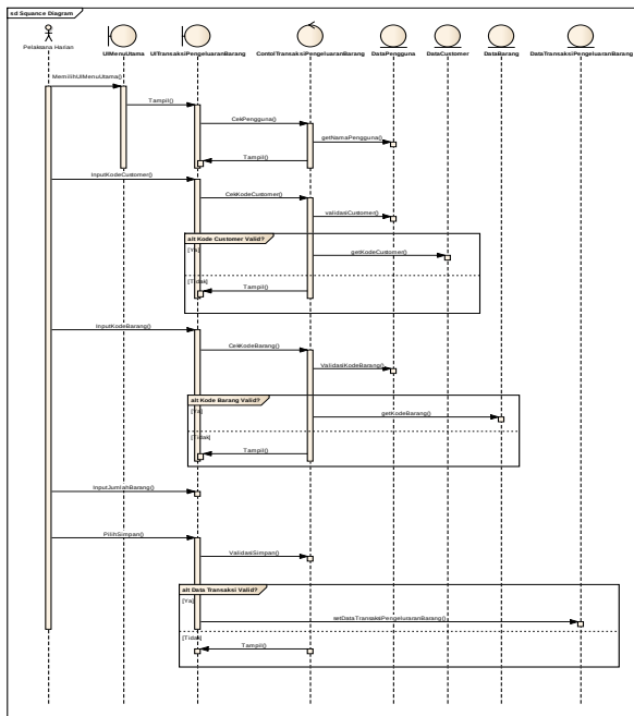
Gambar 11. Sequence Diagram Transaksi Pengeluaran Barang
