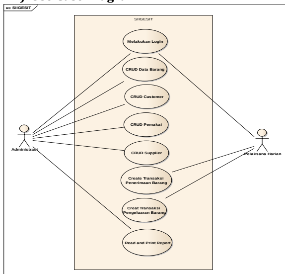
Gambar 1. Use Case Diagram SIIGESIT
