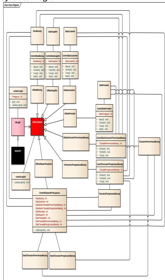
Gambar 10. Class Diagram SIIGESIT
