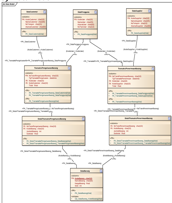
Gambar 12. Data Model SIIGESIT
