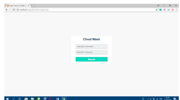
Gambar 5. Halaman Login
