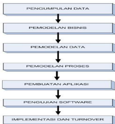
Gambar 2. Tahapan Penelitian
